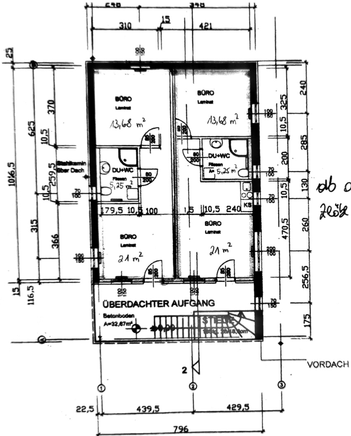
OBERGESCHOSS
